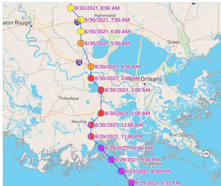
Hurrikan Idas Zugbahn durch Louisiana. Kurz nach dem zweiten Landfall verringerte sich Idas Intensität auf einen Sturm an der Grenze zwischen der 3. und 4. Stärkestufe auf der Saffir-Simpson Skala, das System wurde offiziell aber weiterhin als Kategorie 4 Sturm ausgewiesen. Die Zeitangaben beziehen sich auf europäische Sommerzeit.
